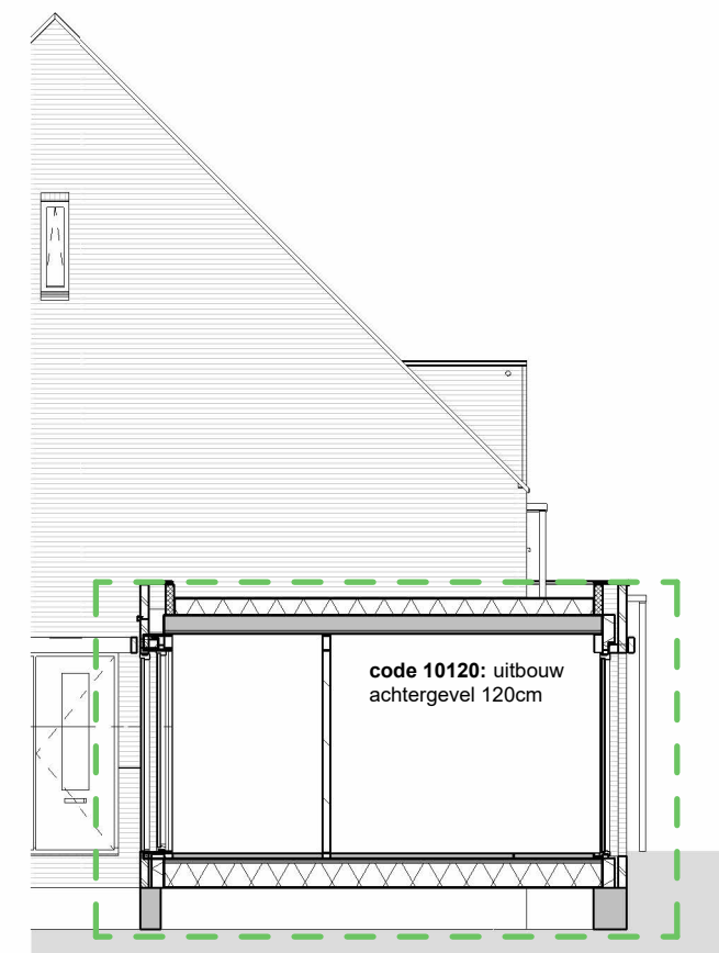
langsdoorsnede
