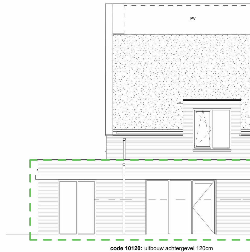
achtergevel
