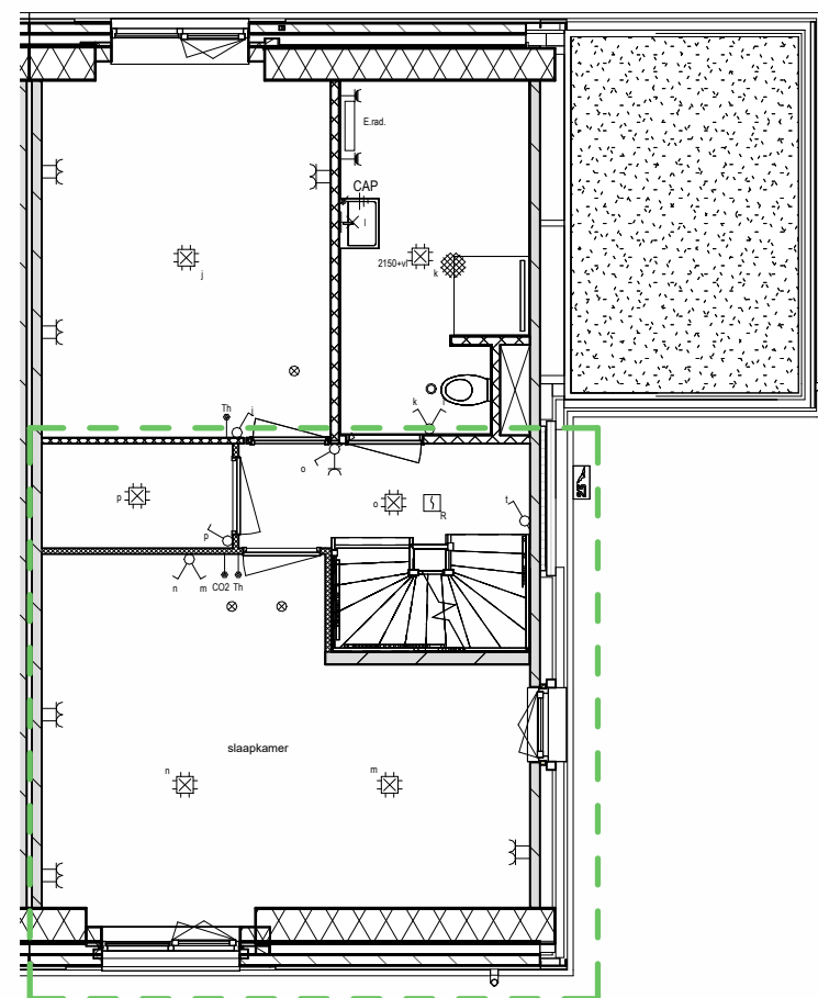
01 eerste verdieping
