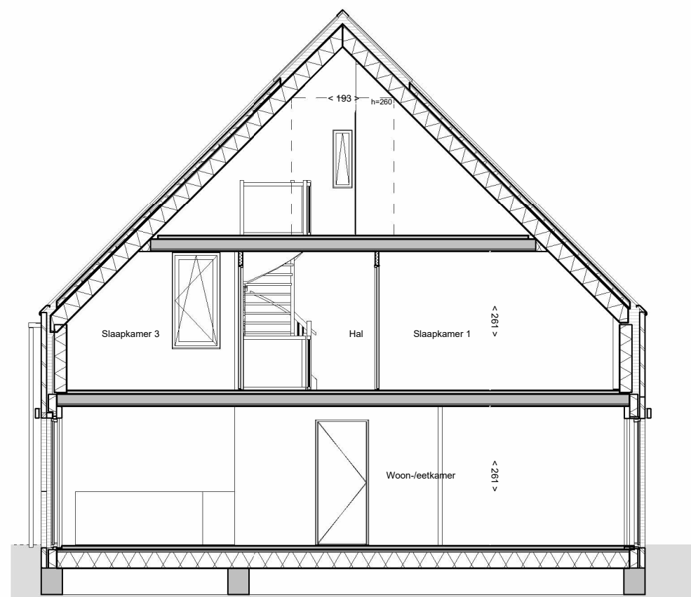
doorsnede B
