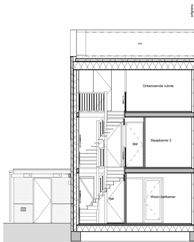
doorsnede A
