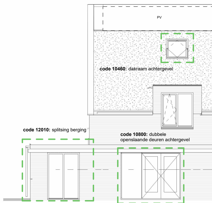
achtergevel
